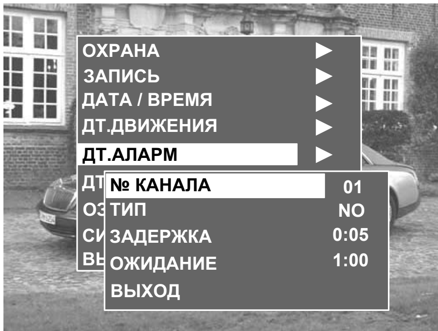
Рис.9. Подменю «ДТ. АЛАРМ».
